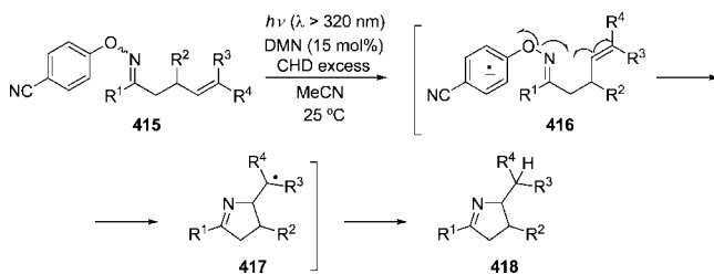
Scheme 170
